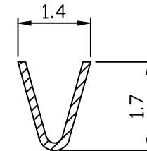
A-A SEC
